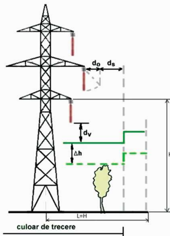
Figura 1.c Profil culoar de trecere LEA 110 kV și zonă împădurită
